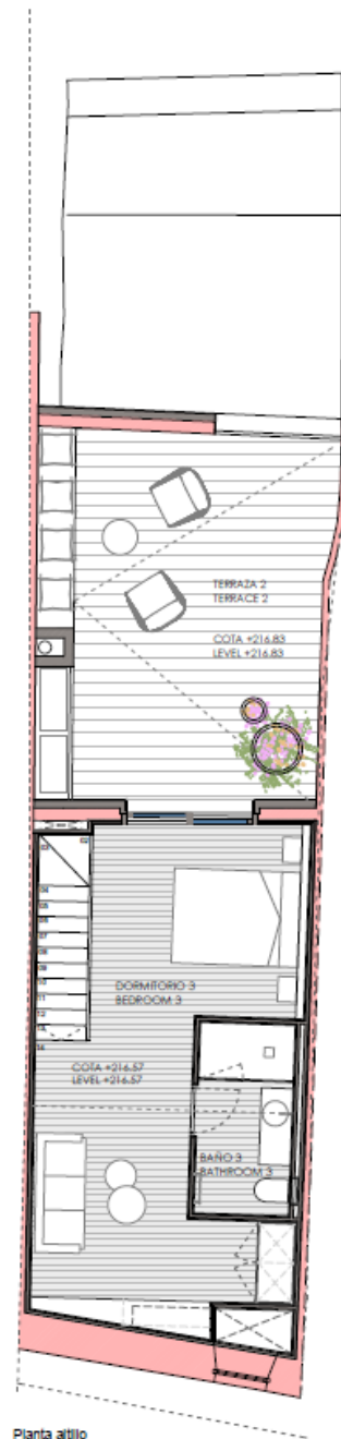
Planta ático
